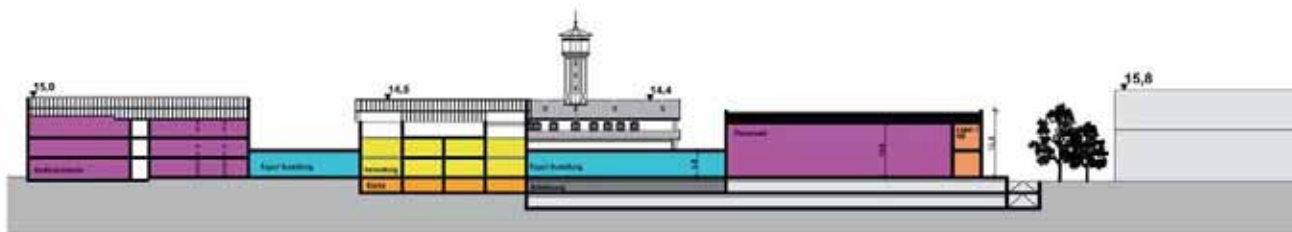
Schnitt A
