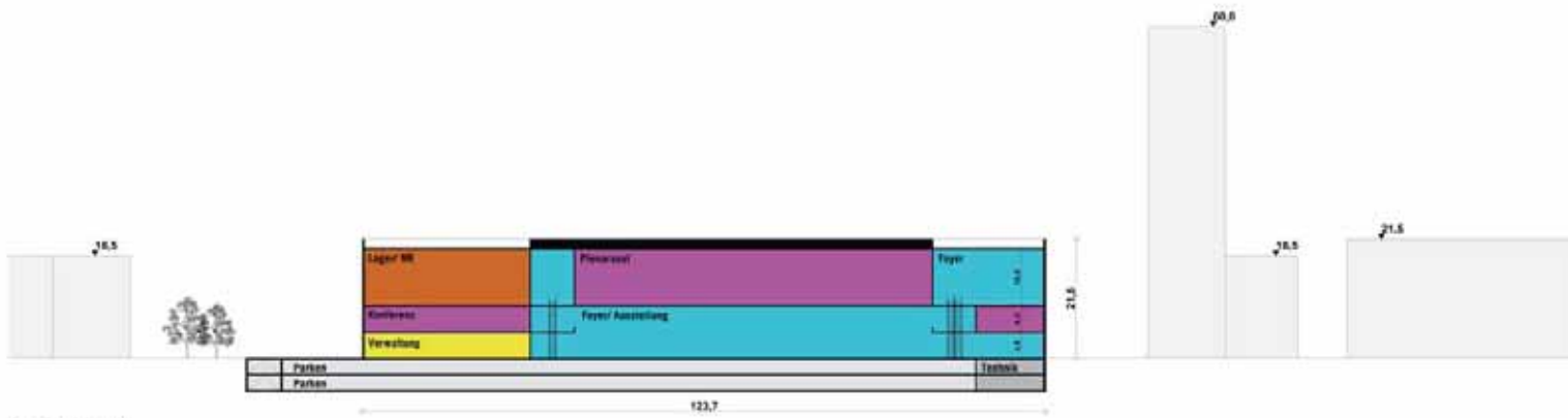
Schnitt A
